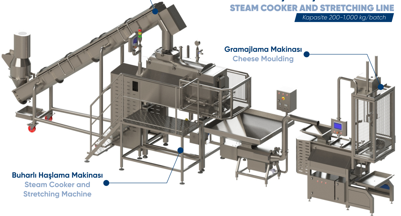
Teleme Konveyörü Curd Conveyor
