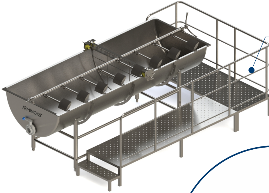
Beyaz Peynir Mayalama Teknesi White Cheese Fermentation Vat
