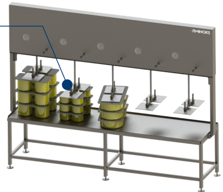
Peynir Presi Cheese Press
